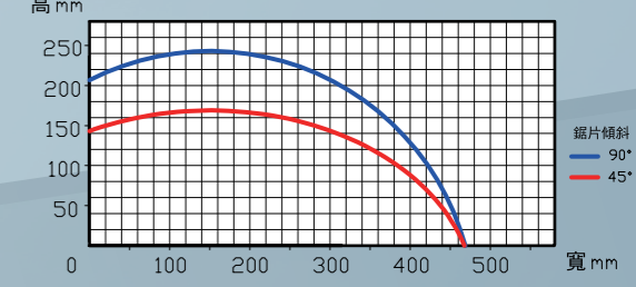
T5/T5S 26" 鋸片-工作台旋轉 45° 時鋸切能力圖
