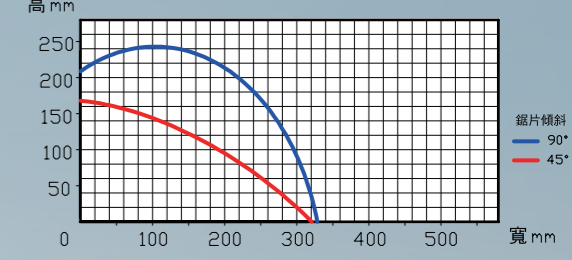
T5/T5S 26" 鋸片-工作台旋轉 67.5° 時鋸切能力圖
