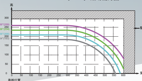
JIH-NC30L : 24吋~30吋 鋸切能力圖
