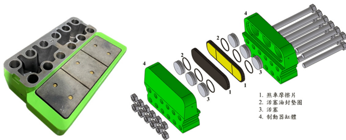
離岸風電轉向系統剎車單元
